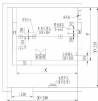
井道平面
