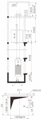
井道立面布置图
