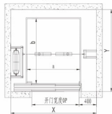
井道平面
